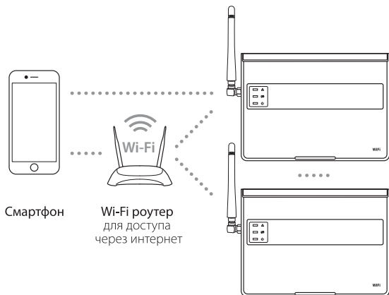
Рис. 4. Схема управления модулями Neptune ProW+ WiFi со смартфона.
